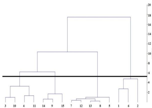
شکل ۱: دندروگرام حاصل از تجزیه خوشه‌ای لاین‌های ذرت در شرایط نرمال
