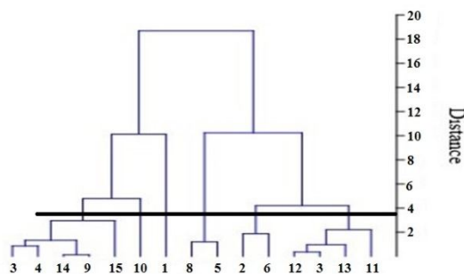
شکل ۳: دندروگرام حاصل از تجزیه خوشه‌ای لاین‌های ذرت بر اساس میانگین صفات در هر دو شرایط
